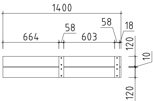
PARAPET 1b - PARAPET 1b
