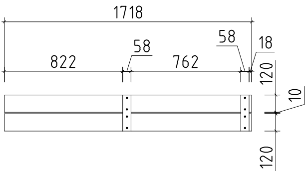
PARAPET 2b - PARAPET 2b
