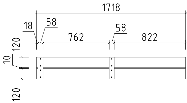
PARAPET 2a - PARAPET 2a
