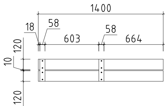
PARAPET 1a - PARAPET 1a
